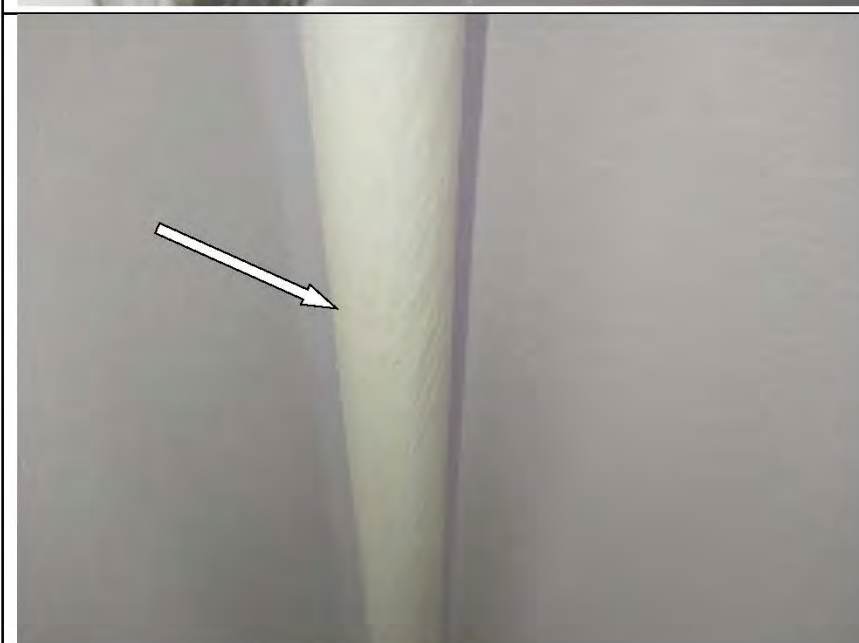
Фото №75. Окрашивание труб отопления выполнено с дефектами в спальне (подтеки)
