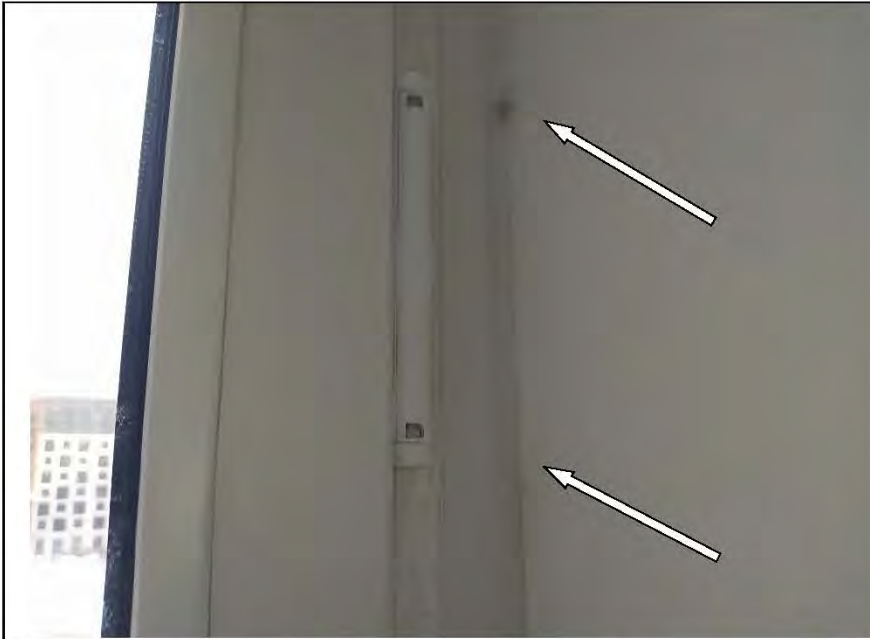
Фото №28. Следы скопления пыли, свидетельствующие об инфильтрации воздуха через петли оконного блока в гостиной.
